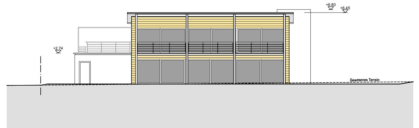
Südfassade
