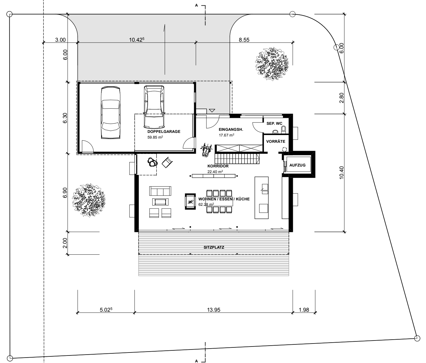
Erdgeschoss
