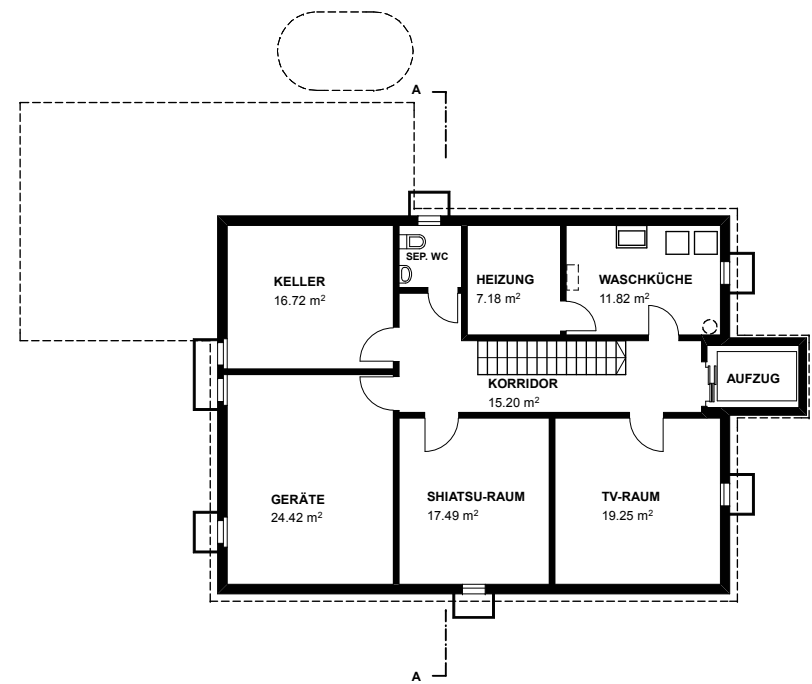
Untergeschoss
