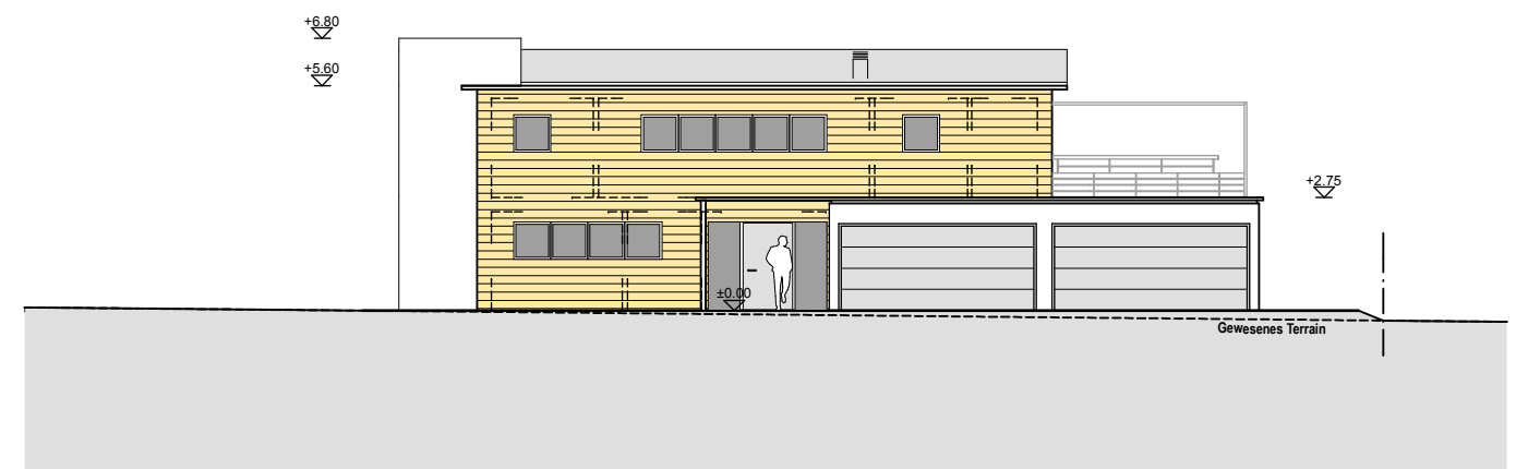
Nordfassade
