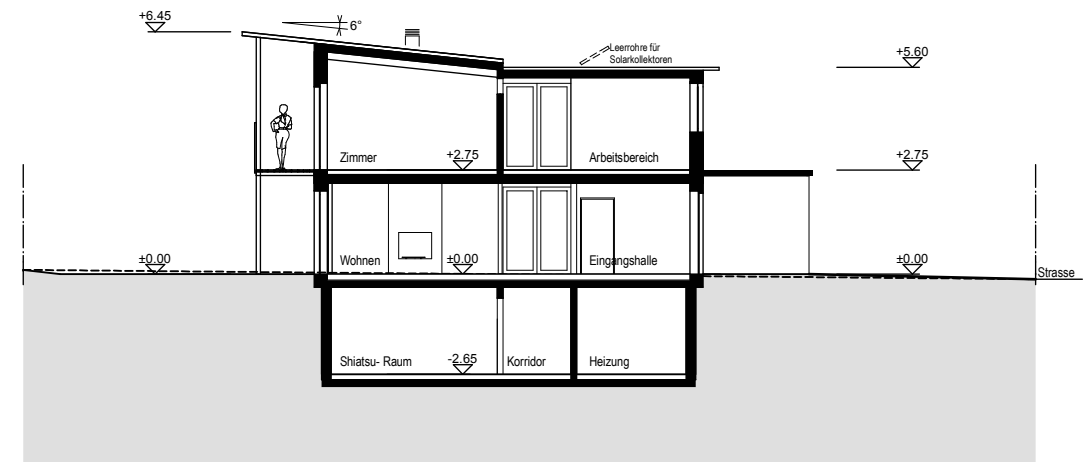
Querschnitt A-A
