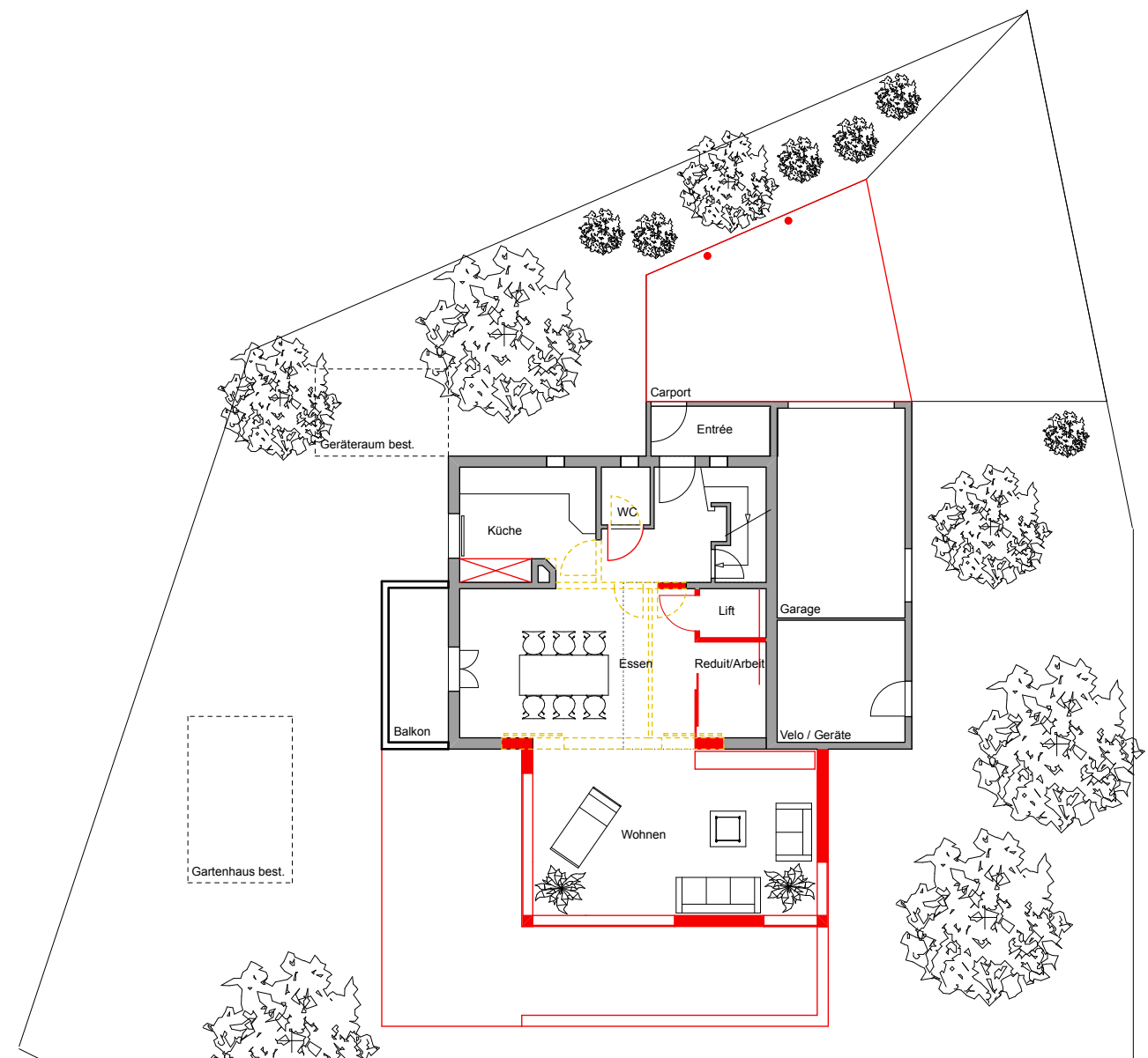
Erdgeschoss
