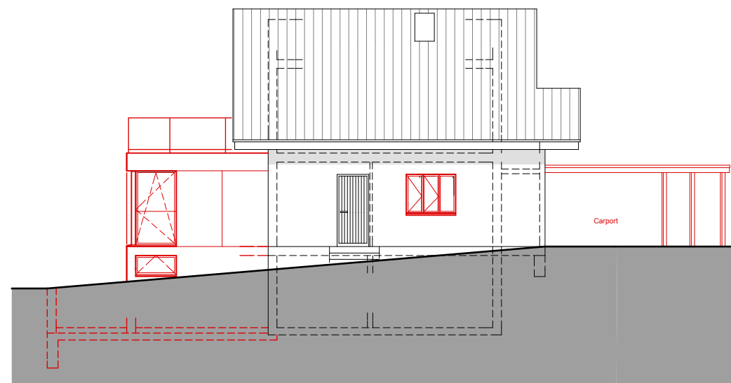
Ostfassade
