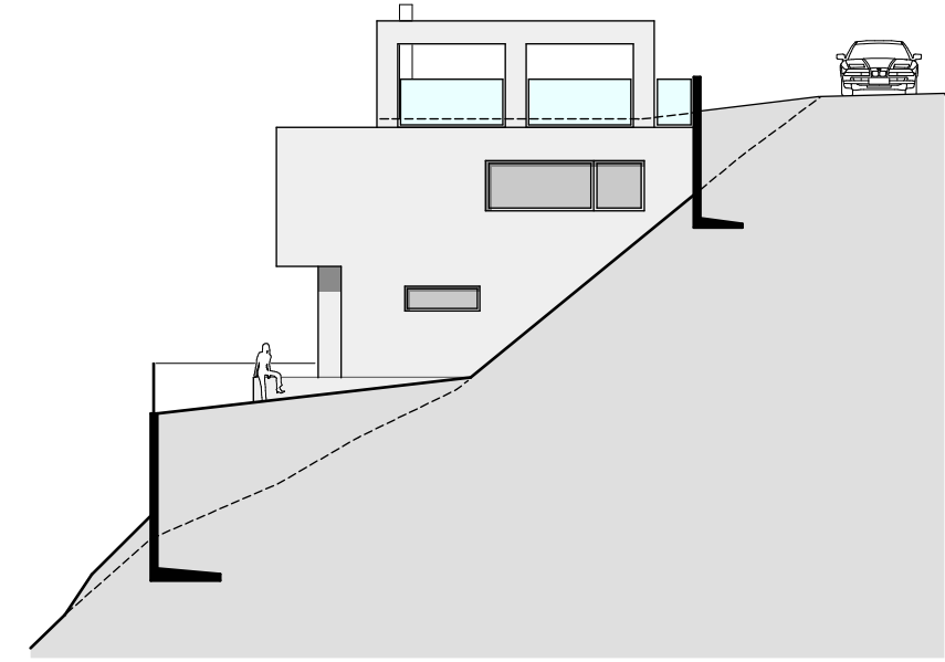
Facciata Est
